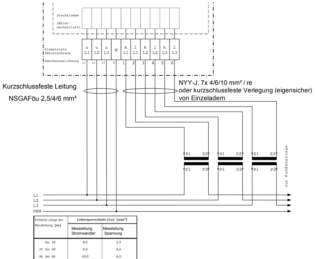
Bild B.3: Beispiel Wandlerverdrahtung für MS-Anlagen mit NS-seitiger Wandlermessung ( \leq 630 kVA)
